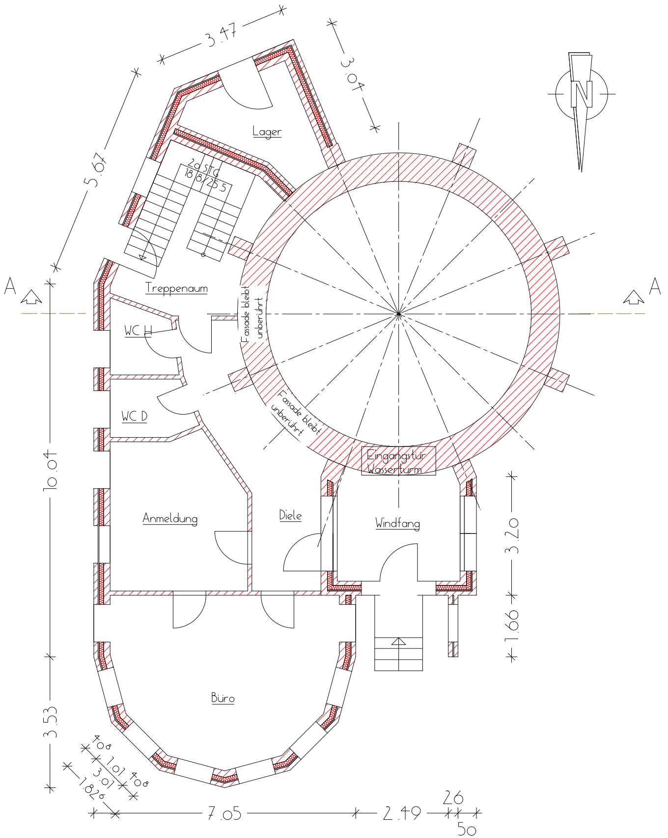
Grundriss Erdgeschoss 1:100
