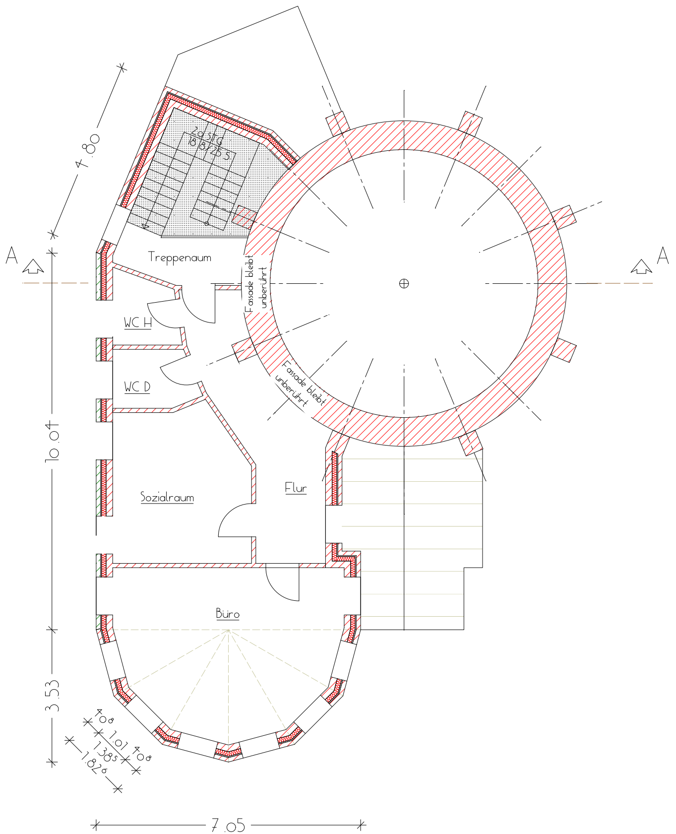
Grundriss Obergeschoss 1: 100
