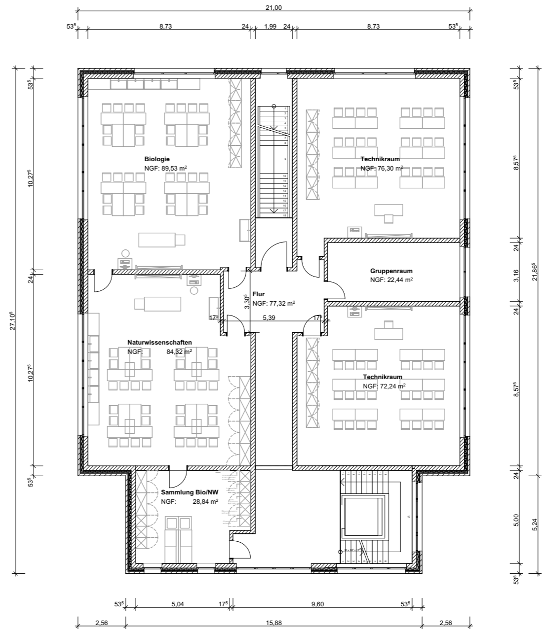
Obergeschoss
