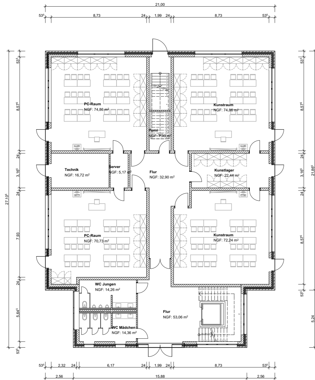
Erdgeschoss
