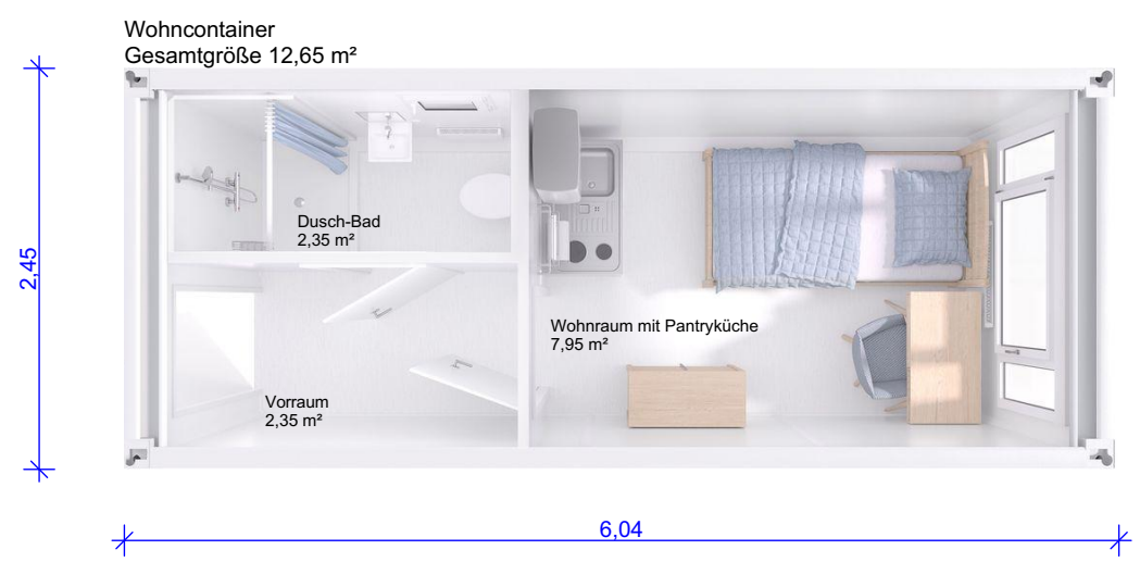
Detailansicht Wohneinheit
