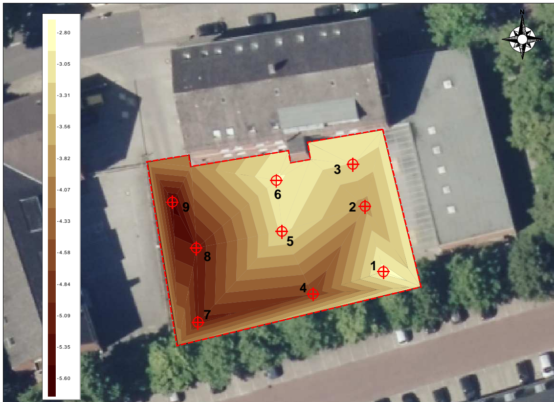
Abb. 2: Auffüllungsmächtigkeiten
